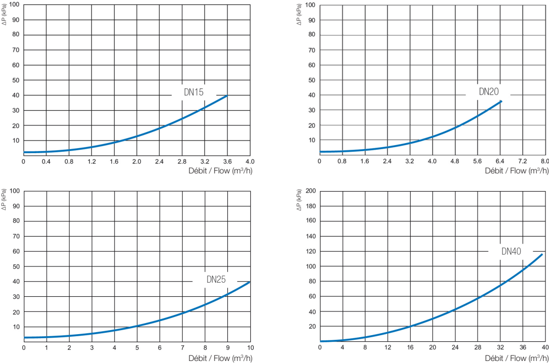
WM - Abaque des pertes de charge
